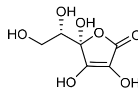
Fig. 1. Vitamin C (L-Ascorbic acid).
